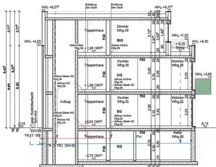
Schnitt B-B, entspricht Hausnr. 138a und Hausnr. 138b
