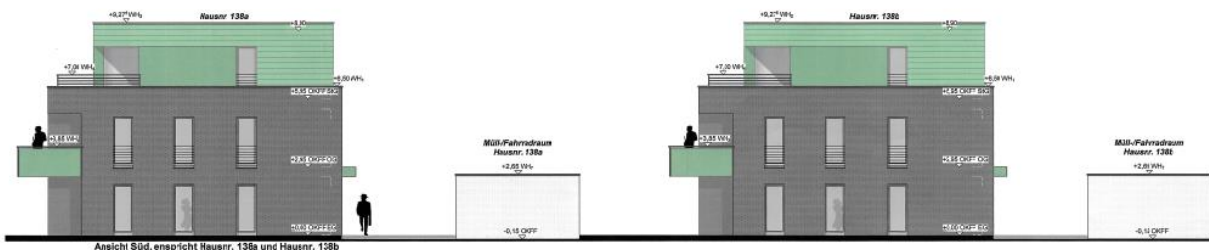
Ansicht Süd, entspricht Hausnr. 138a und Hausnr. 138b
